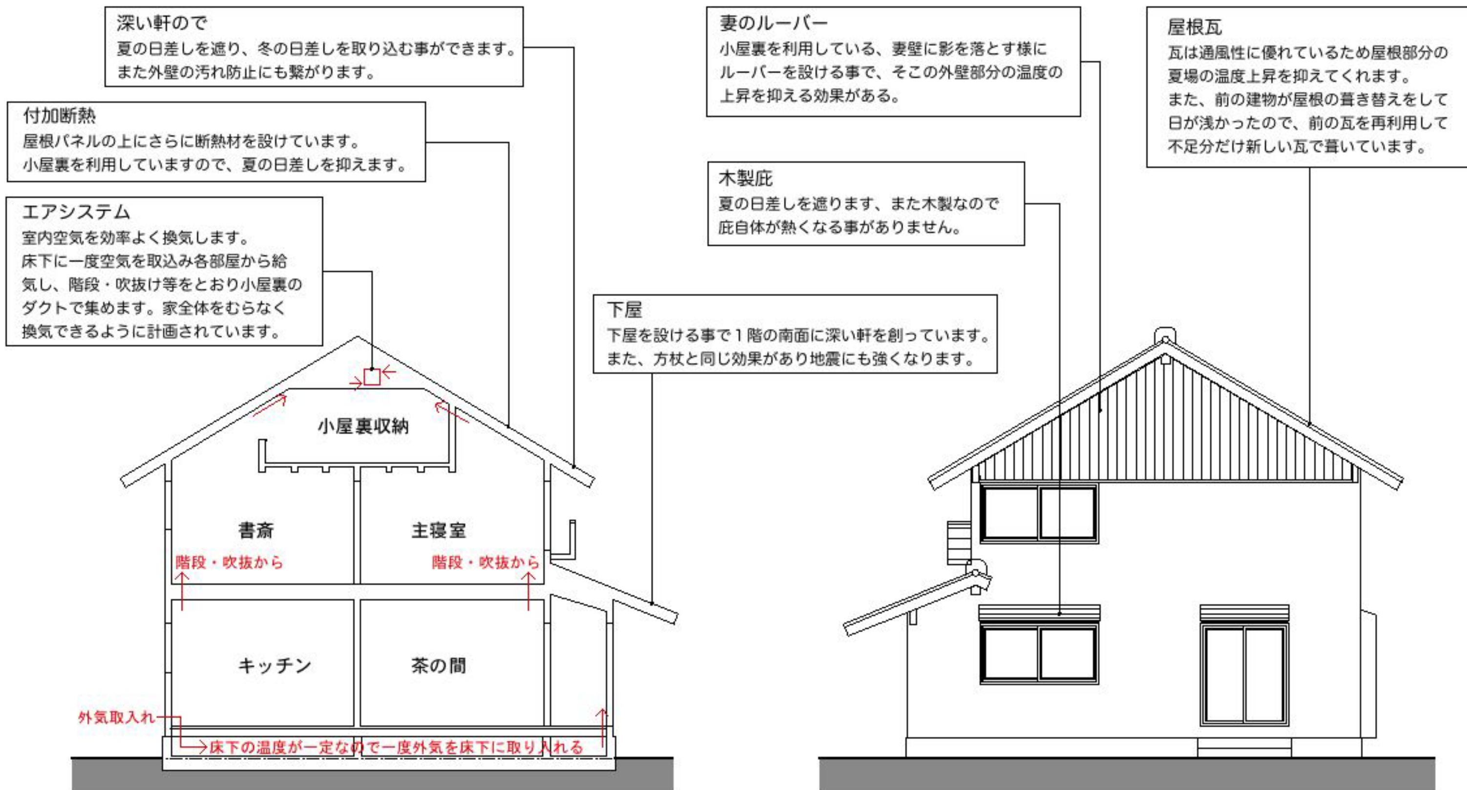
断面図
